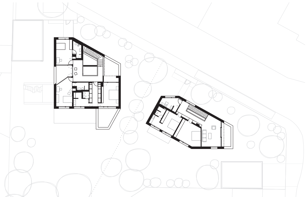
obergeschoss . first floor
